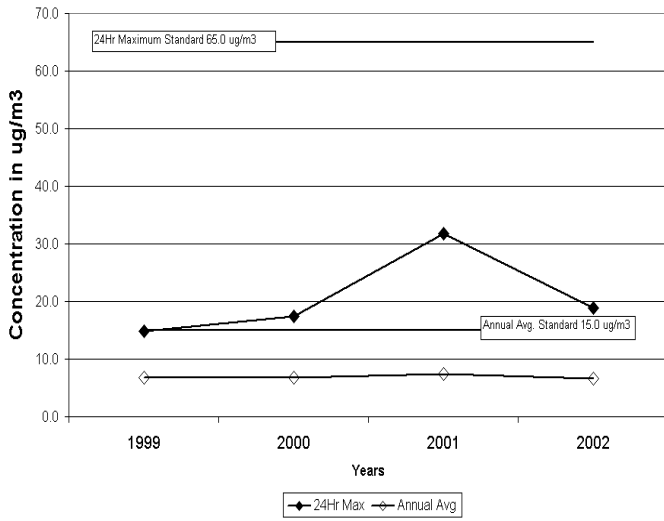
Pueblo - Ambient Trends - PM 2.5
